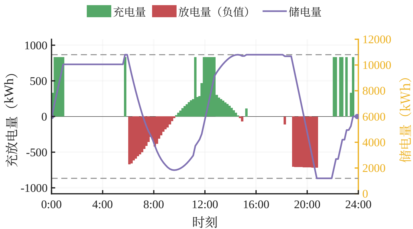
储能充放电与储电量
